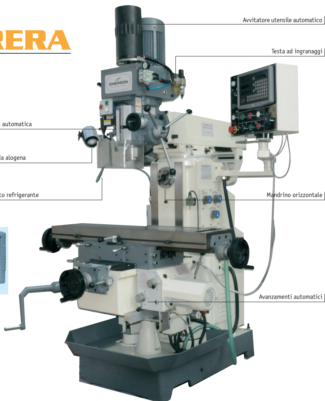
Visualizzatore di quote a tre assi di serie
