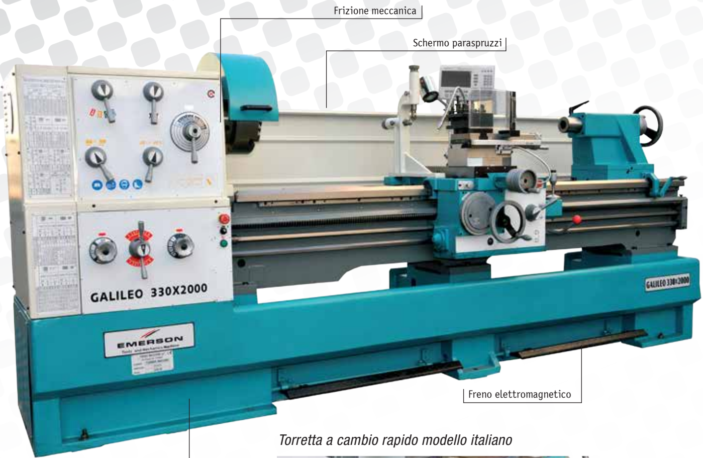
Basamento monolitico in ghisa
